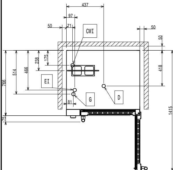
Boven aanzicht
