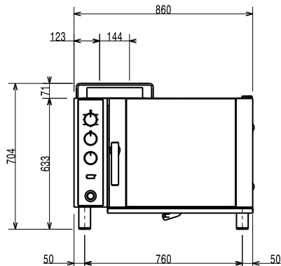
Front aanzicht
